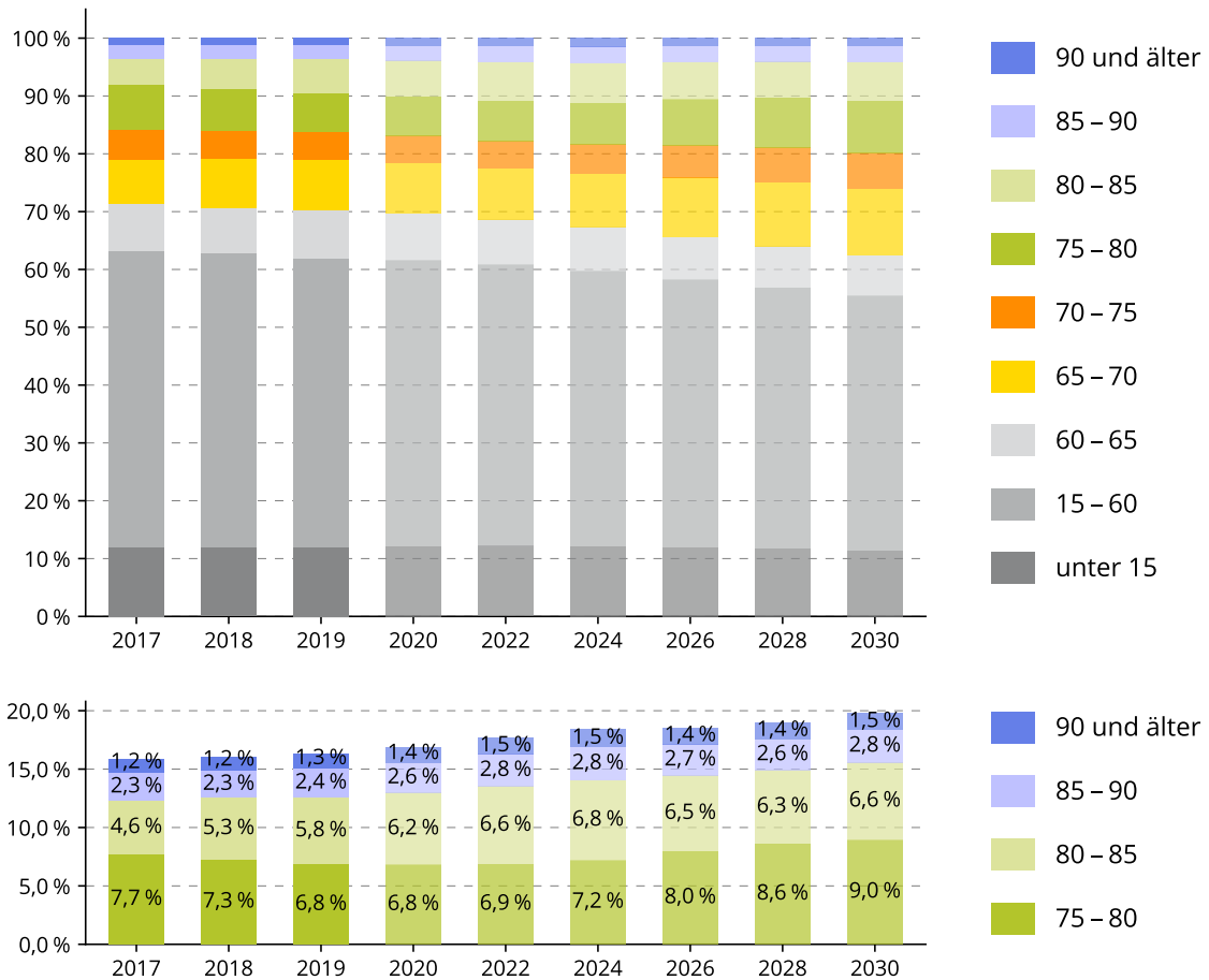
Abbildung 1: oben - Anteil der Altersgruppen an der Gesamtbevölkerung (2017-2030) in der Stadt Senftenberg - relativ (Prozent);
