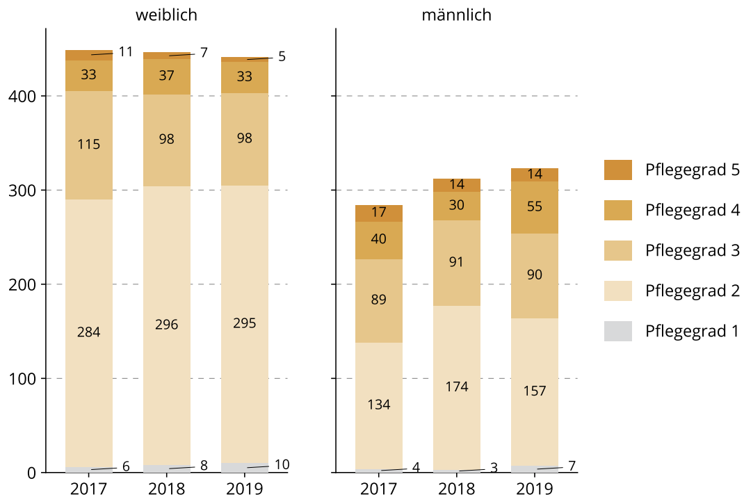
Abbildung 6: Anzahl der Pflegebedürftigen nach Pflegegrad in häuslicher Pflege – Frauen/Männer (2017–2019) in der Stadt Senftenberg – absolut
