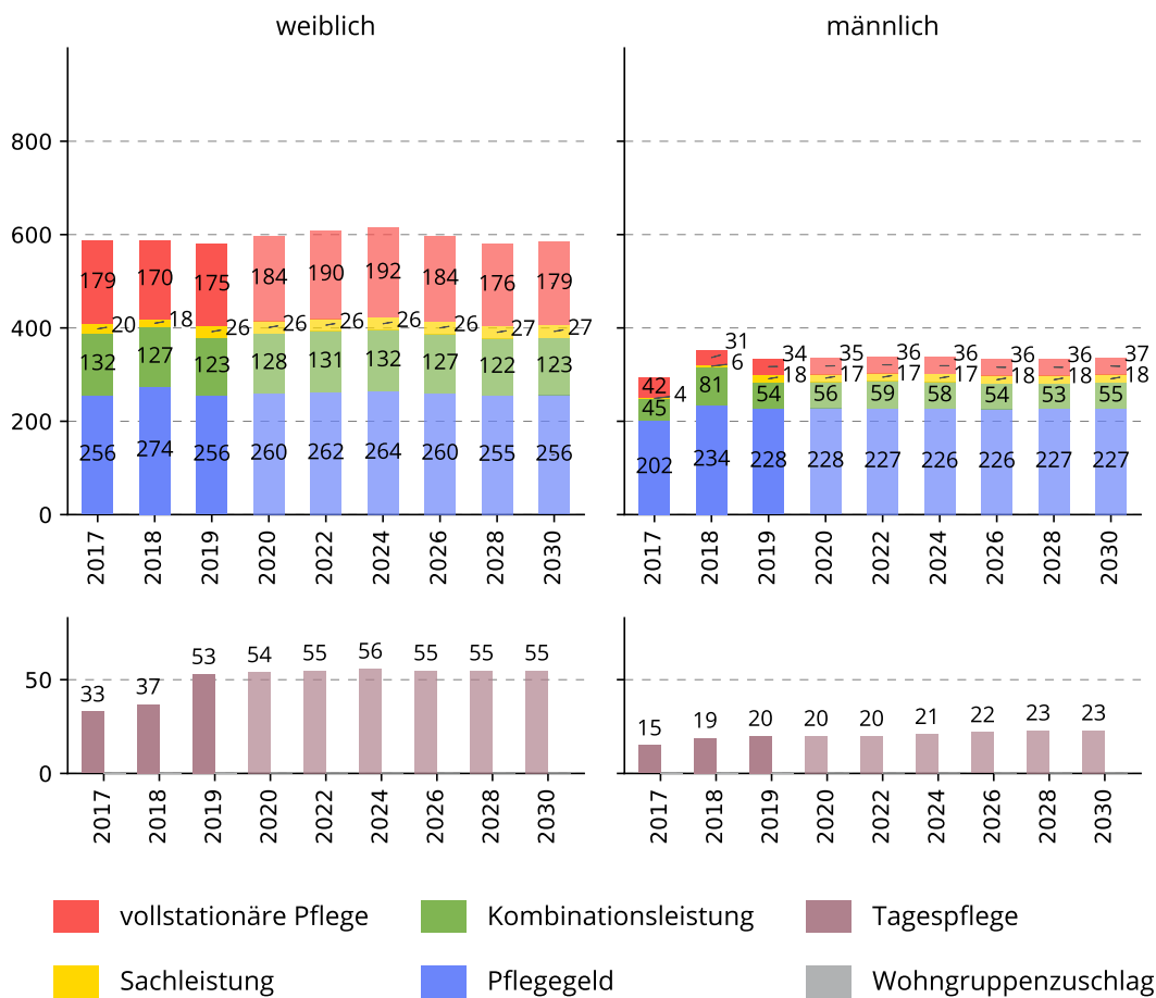
Abbildung 5: Anzahl der Pflegebedürftigen (PG 2-5) nach Art der Versorgung – Frauen/Männer (2017-2030) in der Stadt Senftenberg – absolut
