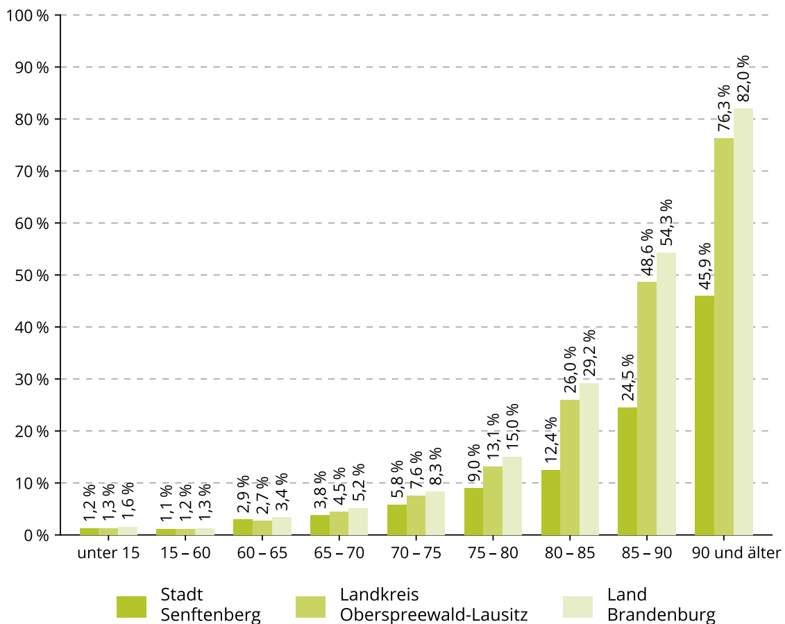
Abbildung 3: Anteil der Pflegebedürftigen an der Bevölkerung nach Alter (2019) in der Stadt Senftenberg – relativ (Prozent); Quelle der Daten zum Landkreis und Land Brandenburg: Brandenburger Pflegedossiers – Analyse der Pflegestatistik 2019 [4]
