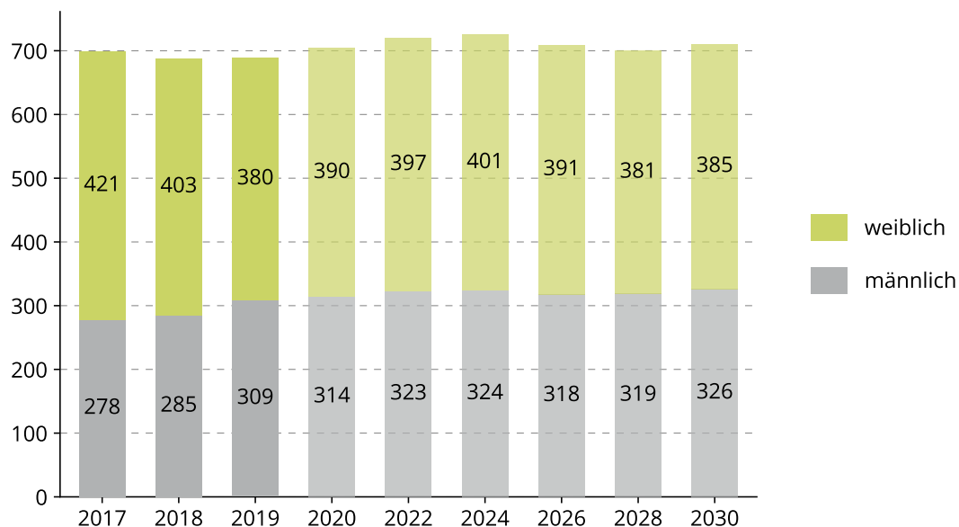
Abbildung 10: Anzahl der demenziell Erkrankten nach Geschlecht im Zeitverlauf (2017–2030) in der Stadt Senftenberg - absolut
