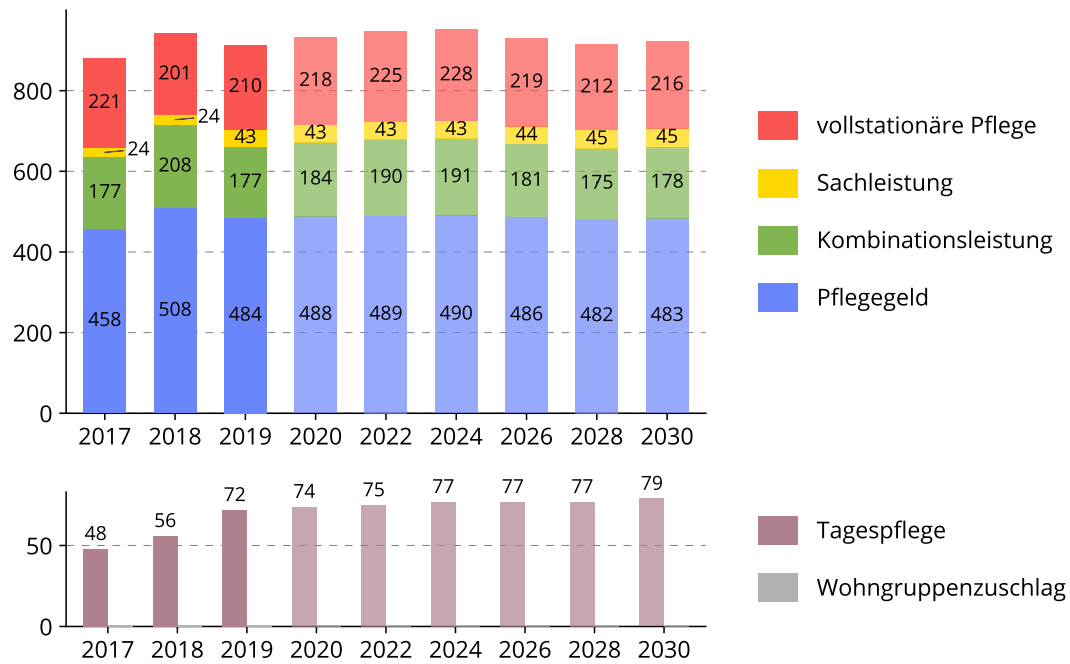
Abbildung 4: Anzahl der Pflegebedürftigen (PG 2-5) nach Art der Versorgung im Zeitverlauf (2017-2030) in der Stadt Senftenberg – absolut
