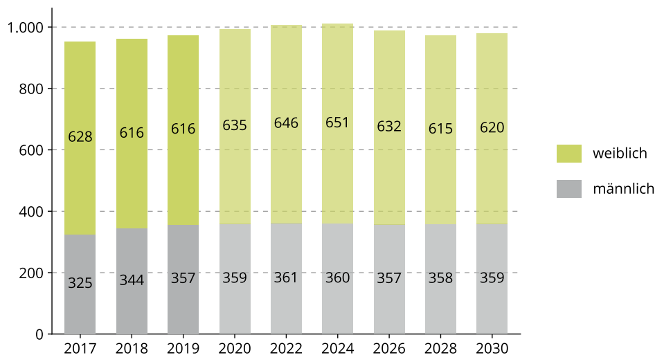
Abbildung 2: Anzahl der Pflegebedürftigen nach Geschlecht im Zeitverlauf (2017–2030) in der Stadt Senftenberg – absolut
